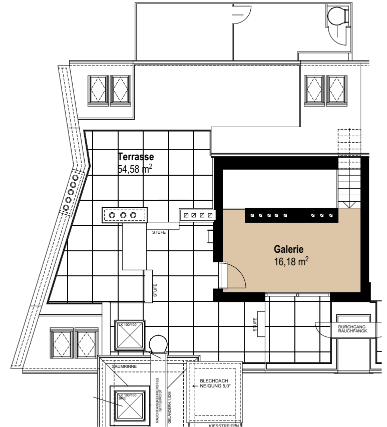
2.DACHGESCHOSS
