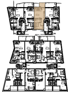
1.DACHGESCHOSS
