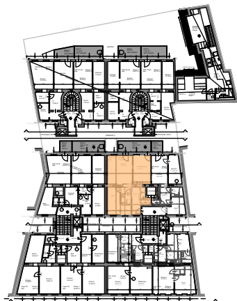
2.OBERGESCHOSS
